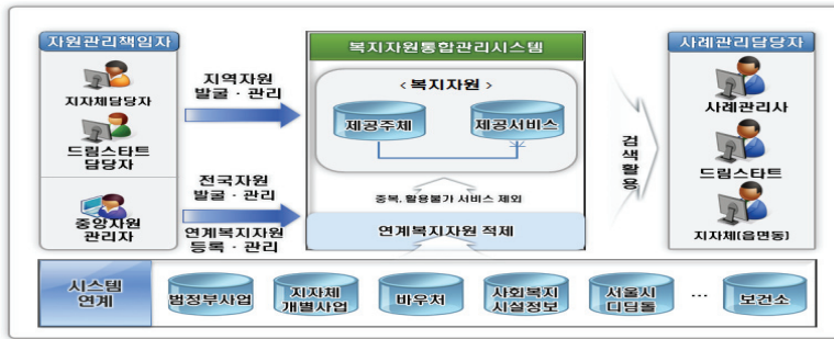
[복지자원통합관리시스템 업무흐름도]
