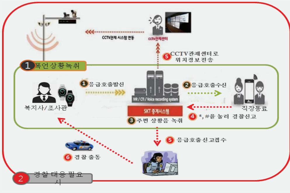
〈 안전지킴이 구성도 〉
